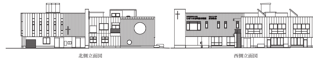
北側立面図
